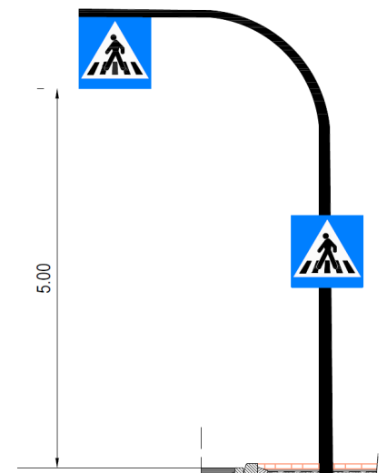
COUPE DE PRINCIPE POTEAU DE SIGNALISATION
